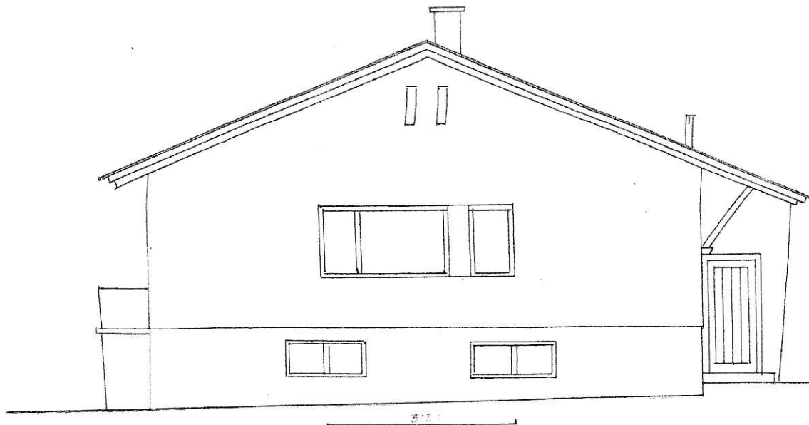
NORDGIEBEL 1:100
